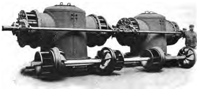
Fig. 38. Kitzende Drosselturbine mit vier Laufrädern.
